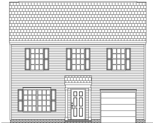
Elevation A
